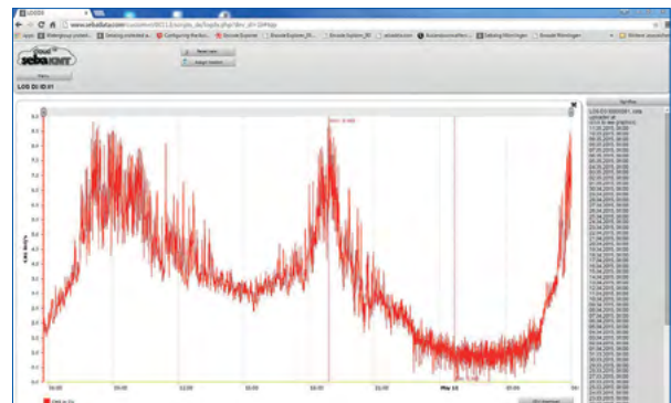
Control del flujo en línea con datos del aparato de medición ultrasónica SebaFlow
